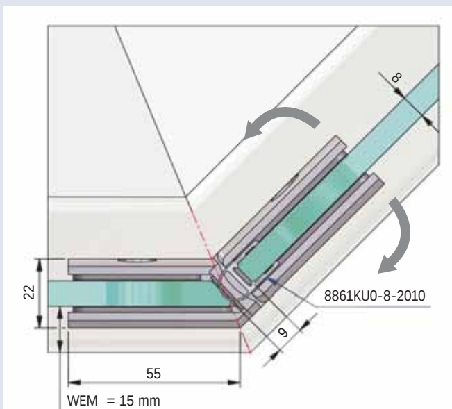
Türflügel einseitig 90° öffnend/wing of the door opens in one direction 90°
