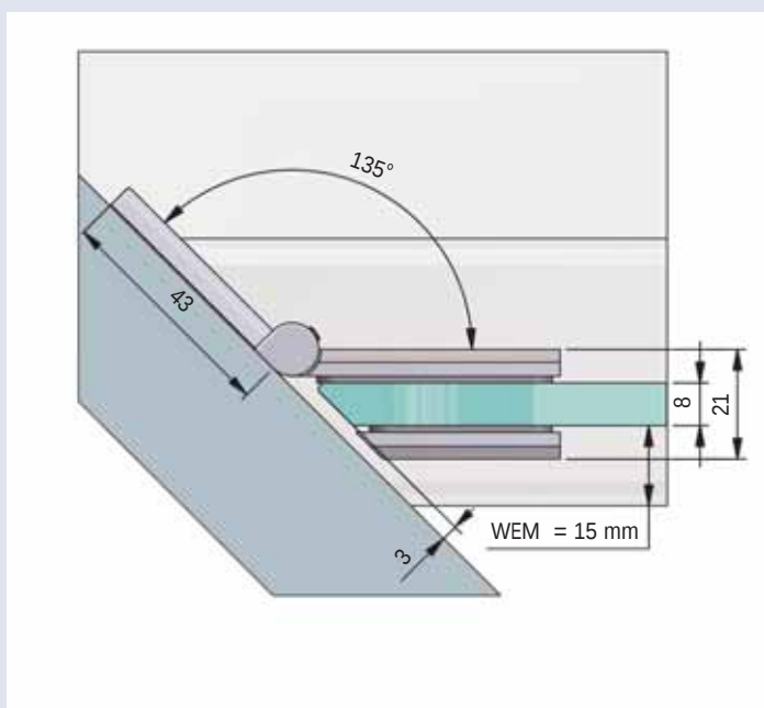
Glasbearbeitung für Winkelverbinder 8427MS bei 135°, Bei anderen Gradzahlen ändert sich der Gehrungswinkel dementsprechend./ Glass processing for corner bracket 8427MS at 135°, with other angles the miter angle is changing accordingly.
