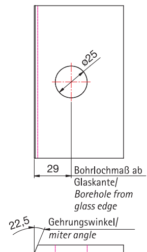
Glasbearbeitung für Winkelverbinder 8425MS bei 135°, Bei anderen Gradzahlen ändert sich der Gehrungswinkel wie in folgender Tabelle beschrieben./ Glass processing for corner bracket 8425MS at 135°, with other angles the miter angle is changing, Please use the follow- ing table when applying other angles.
