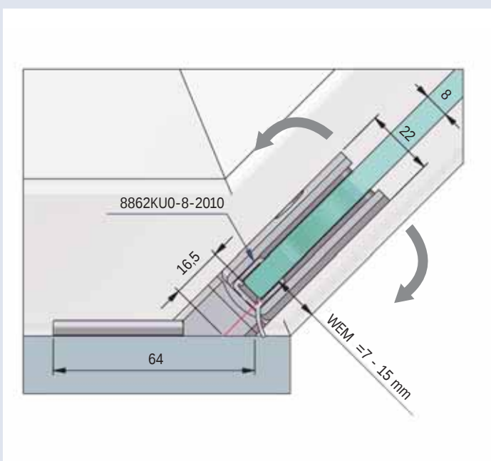
Glasbearbeitung mit Dichtprofil/ Glass processing with sealing profile Art.-Nr. 8862KU0-8-2010
