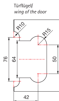
Glasbearbeitung ohne Dichtprofil/ Glass processing without sealing profile
