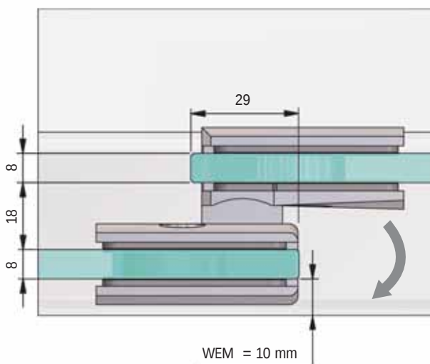
Türflügel nach außen hin 180° öffnend/wing of the door only opening outward 180°
