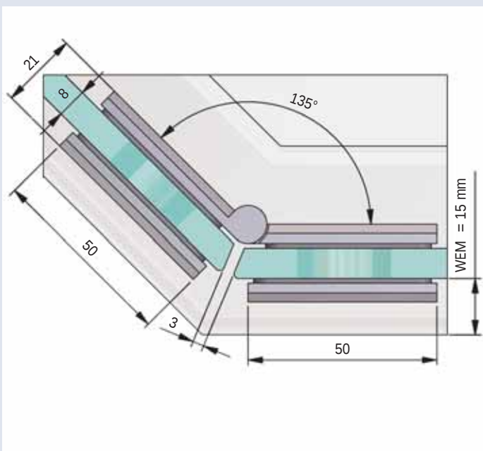
Glasbearbeitung für Winkelverbinder 8425MS bei 135°, Bei anderen Gradzahlen ändert sich der Gehrungswinkel wie in folgender Tabelle beschrieben./ Glass processing for corner bracket 8425MS at 135°, with other angles the miter angle is changing, Please use the follow- ing table when applying other angles.
