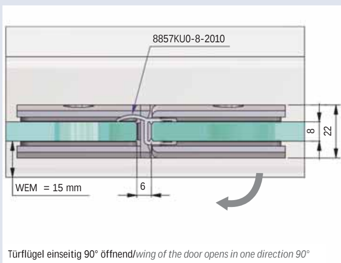
Glasbearbeitung mit Dichtprofil/ Glass processing with sealing profile Art.-Nr. 8857KU0-8-2010
