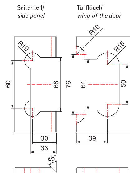
Glasbearbeitung ohne Dichtprofil/ Glass processing without sealing profile
