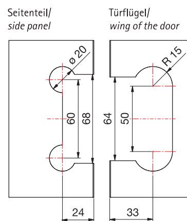
Glasbearbeitung mit Dichtprofil/ Glass processing with sealing profile Art.-Nr. 8861KU0-8-2010
