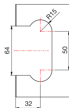
Türflügel/ wing of the door
