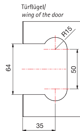
Glasbearbeitung mit Dichtprofil/Glass processing with sealing profile Art.-Nr. 8861KU0-8-2010
