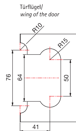
Glasbearbeitung mit Dichtprofil/ Glass processing with sealing profile Art.-Nr. 8861KU0-8-2010
