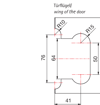
Glasbearbeitung ohne Dichtprofil/ Glass processing without sealing profile
