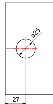
Glasbearbeitung für Längsverbinder 8428MS bei bündiger Wandmontierung/ Glass processing for Inline connector 8428MS flush in-wall application
