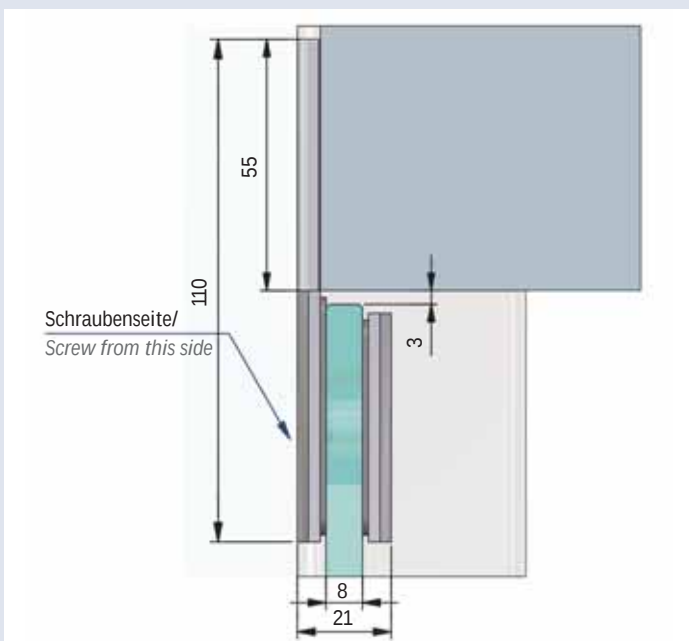
Glasbearbeitung für Längsverbinder 8428MS bei bündiger Wandmontierung/ Glass processing for Inline connector 8428MS flush in-wall application
