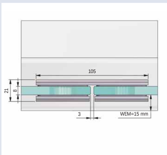
Glasbearbeitung für Längsverbinder 8422MS / Glass processing for Inline connector 8422MS
