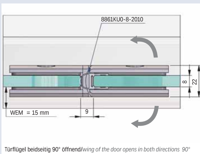
Glasbearbeitung mit Dichtprofil/ Glass processing with sealing profile Art.-Nr. 8861KU0-8-2010
