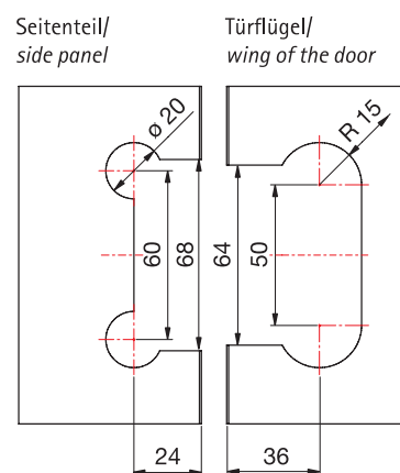
Glasbearbeitung mit Dichtprofil/ Glass processing with sealing profile Art.-Nr. 8857KU0-8-2010
