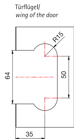
Glasbearbeitung mit Dichtprofil/ Glass processing with sealing profile Art.-Nr. 8861KU0-8-2010
