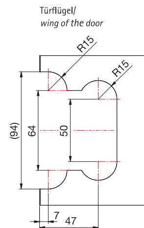
Glasbearbeitung ohne Dichtprofil/ Glass processing without sealing profile
