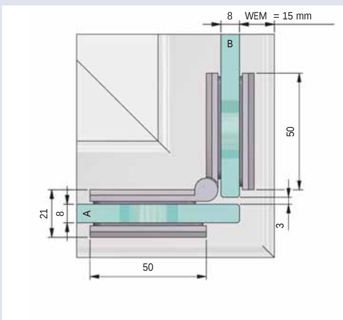
Glasbearbeitung für Winkelverbinder 8421MS/ Glass processing for corner bracket 8421MS
