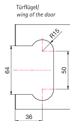
Glasbearbeitung mit Dichtprofil/ Glass processing with sealing profile Art.-Nr. 8857KU0-8-2010
