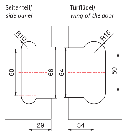
Glasbearbeitung mit Dichtprofil/ Glass processing with sealing profile Art.-Nr. 8861KU0-8-2010
