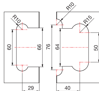
Seitenteil/ side panel
