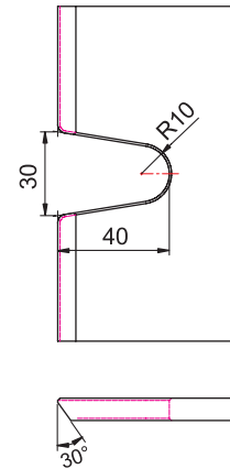
Randausschnitt R40/ edge cutout R40
