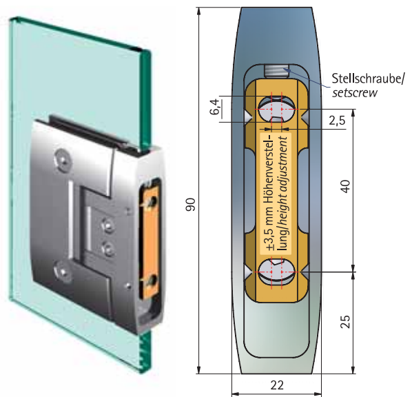
Duschtürpendelband Glas-Wand 90°, 7 mm höhenverstellbar/ Shower door swing hinge; glass-wall, 90°, 7 mm height adjustably Art-Nr.: 8404MS
