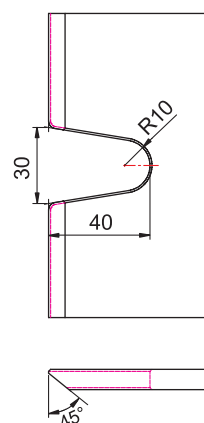
Glasbearbeitung für Winkelverbinder 8427MS bei 135°, Bei anderen Gradzahlen ändert sich der Gehrungswinkel dementsprechend./ Glass processing for corner bracket 8427MS at 135°, with other angles the miter angle is changing accordingly.
